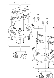
ETB-010164, Tarcza do rozśiewu granicznego TS 5-9
