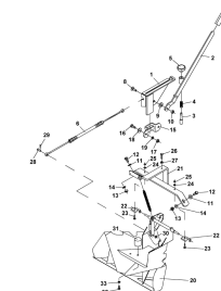
ETB-010168, Ekran rozśiewu granicznego z obu str. Ciężno Bowdena ze zdalnym sterowaniem
