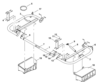
ETB-010173, Rurowy pałąk ochronny składany i trymer
