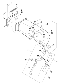
ETB-010206, Lejek odchylany do urządzenia rozsiewającego R8
