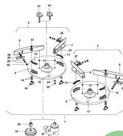
ETB-010162, Tarcza rozśiewająca OS 20-28 / HSS
