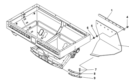
ETB-010200, Osłona przeciwbłotna
