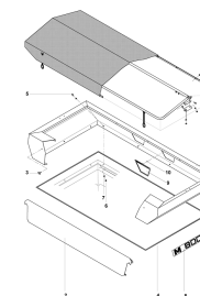
ETB-010196, Nadstawka nad zbiornik M 800
