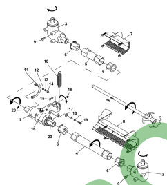
ETB-010174, Napęd ZA-ML
