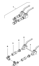
ETB-010187, Siłownik hydrauliczny pojedynczej zasuw jednostronnego działania
