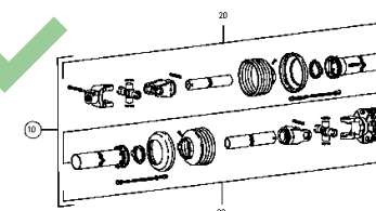
ETB-010208, Wałki przekładnikowe Walterscheid
