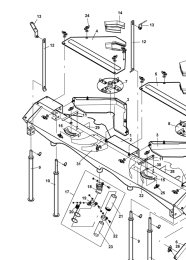
ETB-010204, Lejek środkowy do urządzenia rozsiewającego R4, R6, R8
