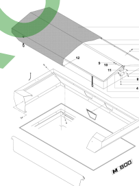
ETB-010199, Składana plandeka M
