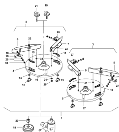
ETB-010161, Tarcza rozśiewająca OS 10-18 / HSS
