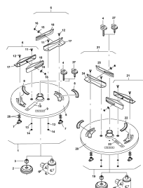
ETB-010165, Tarcza do rozśiewu granicznego TS 10-14
