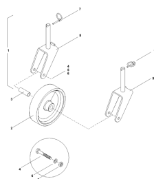
ETB-010201, Urządzenie transportowe i postojowe
