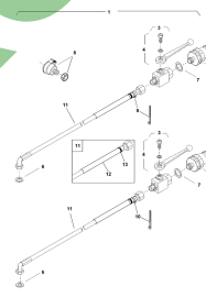
ETB-010187, Siłownik hydrauliczny pojedynczej zasuw jednostronnego działania
