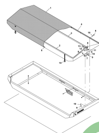
ETB-010198, Składana plandeka L
