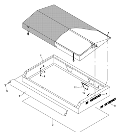
ETB-010193, Nadstawka nad zbiornik N 1800 / N 2300
