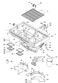
ETB-010157, Rama ze zbiornikiem
