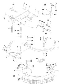
ETB-010170, Zespół do rozsiewu granicznego, lewy „limiter M”
