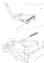
ETB-010175, Przekładnia wejściowa i specjalna przekładnia wejściowa
