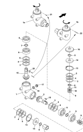
ETB-010176, Przekładnia kątowna
