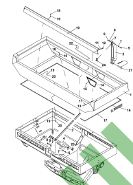
ETB-010195, Nadstawka nad zbiornik L 3000
