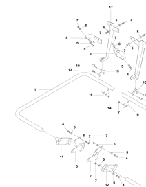
ETB-010172, Rurowy pałąk ochronny odchylany
