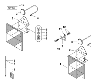
ETB-010203, Oświetlenie przednie
