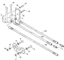
ETB-010189, Zespół dwudrogowy
