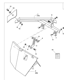
ETB-010167, Ekran rozśiewu granicznego mechaniczny
