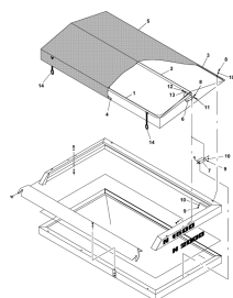
ETB-010197, Składana plandeka N
