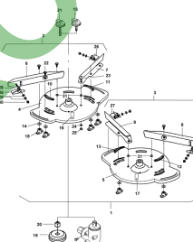
ETB-010163, Tarcza rozśiewająca OS 30-36 / HSS
