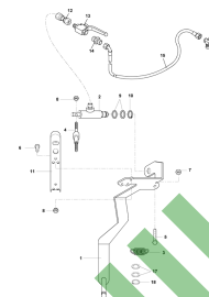
ETB-010171, Automatyczna redukcja dawki
