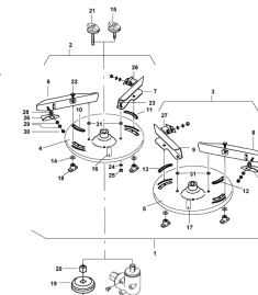
ETB-010160, Tarcza rozśiewająca OS 10-12
